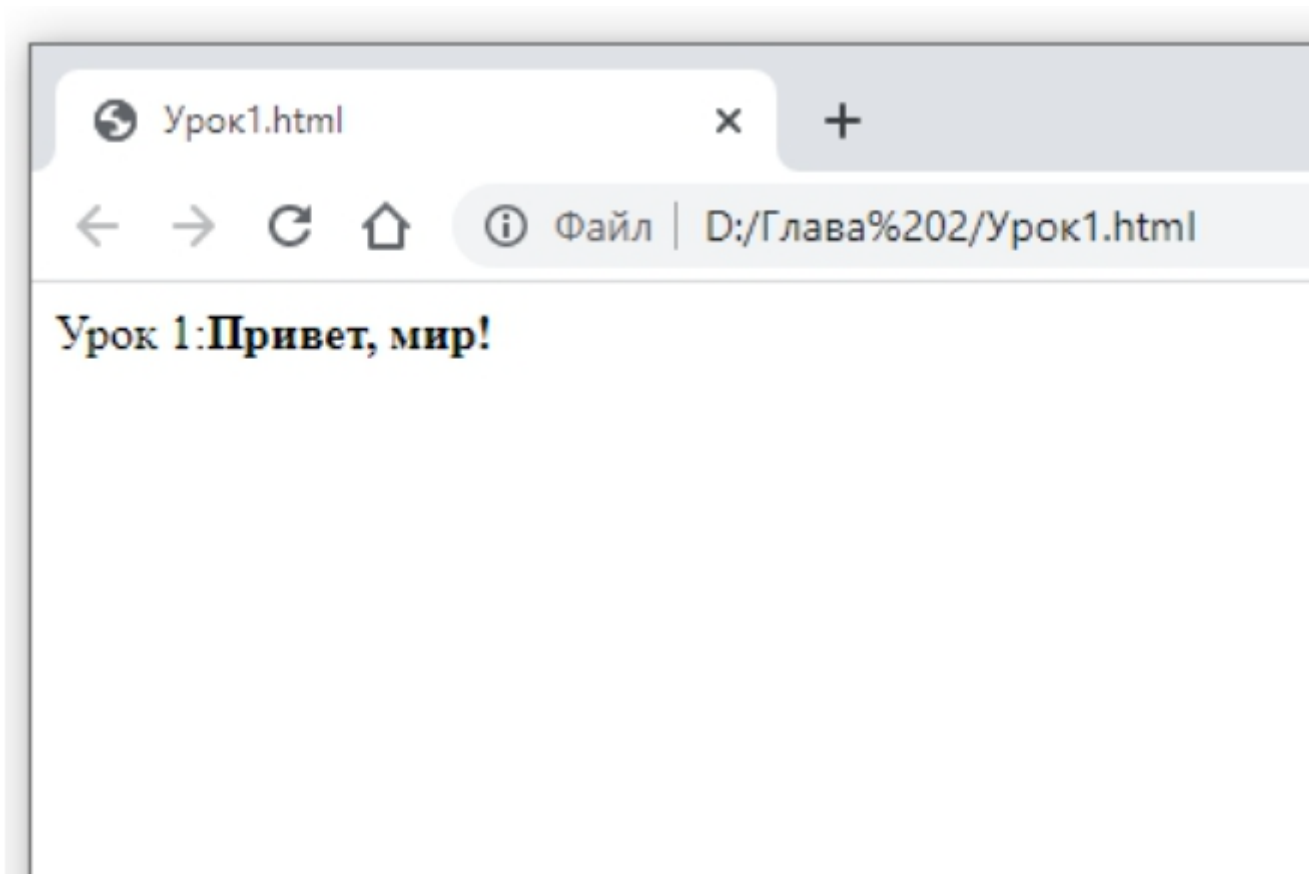
Рисунок 2. Вложенные теги.
